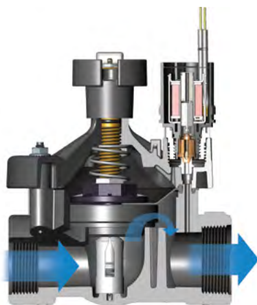
Spaccato PESB
