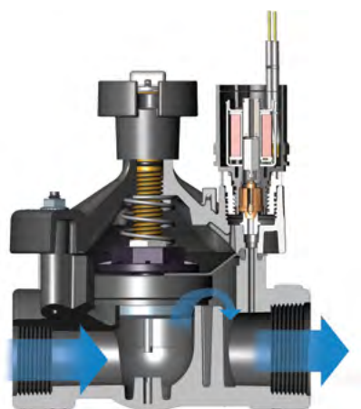
Spaccato PEB
